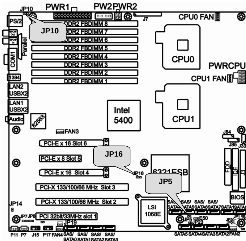
JP5: SAS Enable/Disable jumper
